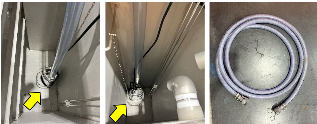
給水ポンプ(左)、排水ポンプ(中)、排水ホース例(右)
