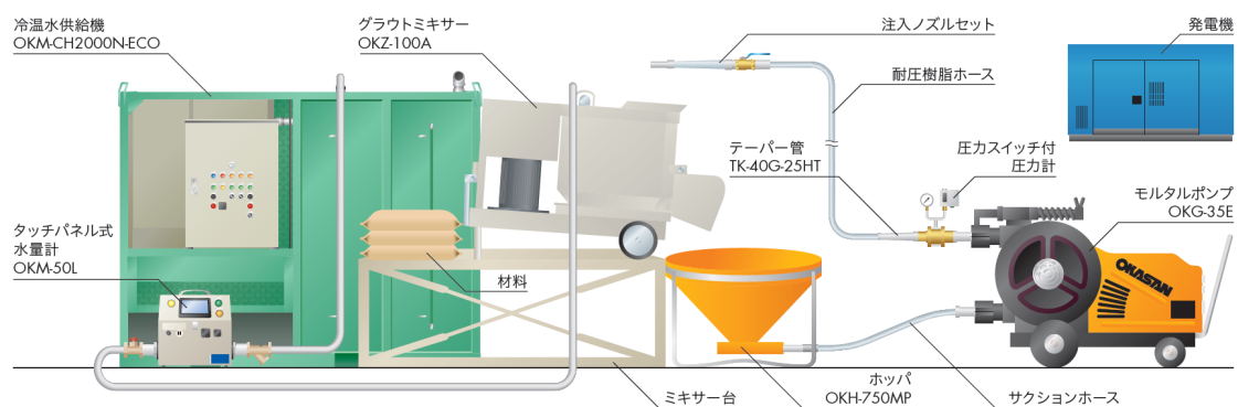
OKM-CHN /OKM-50L を使用したシステム例
