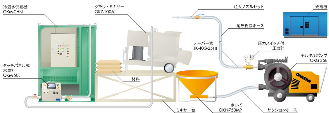
OKM-CHN /OKM-50L を使用したシステム例
